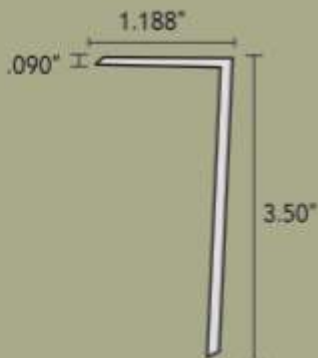
L-MOLDING
