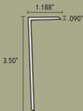
L-MOLDING
